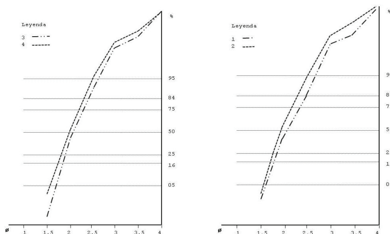
Gráfico 1. Curvas granulométricas de las muestras de los puntos 1, 2, 3 y 4 de la Bahía de Macama
