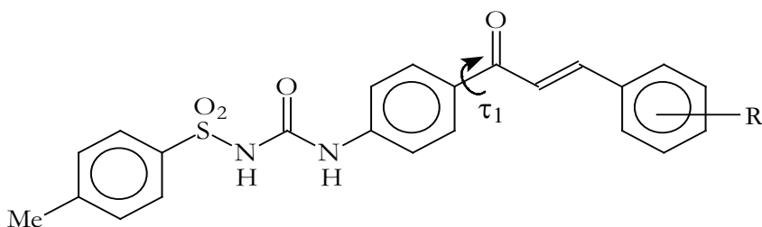
Figura 1. Ángulo rotatable t_1 analizado para las E -1-[4'-(3(sustituido)acrilóil)fenil]-3-tosilureas (a-n)
