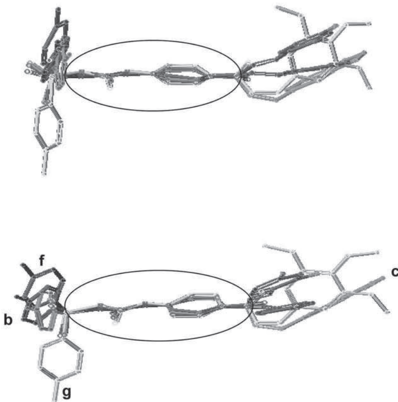
Figura 3. Superposición de las E -1-[4'-(3-(sustituido)acriloil)fenil]-3-tosilureas más activas b , c , f y g . En la región comprendida entre el carbono carbonilo de la chalcona y el átomo de azufre del grupo sulfonilo, se destaca con círculos la clara superposición y coplanaridad entre los átomos.
