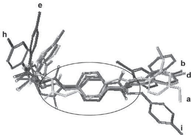
Figura 4. Superposición de las E -1-[4'-(3-(sustituido)acrilóil)fenil]-3-tosilureas menos activas a , d , e , h y i respecto al derivado activo b . A diferencia de lo observado en la figura 11, en la región comprendida entre el carbono carbonilo de la chalcona y el átomo de azufre del grupo sulfonilo (destacada con círculos), no se observa superposición alguna entre los átomos, con excepción del compuesto d que mostró una buena alineación con respecto al compuesto biológicamente activo b .
