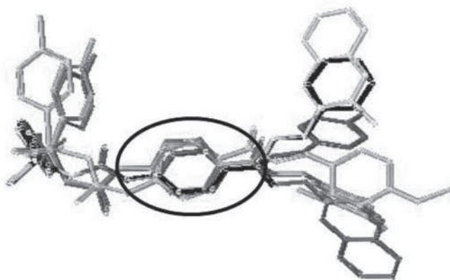
Figura 5. Vistas de la superposición de las E -1-[4'-(3-(sustituido)acrilóil)fenil]-3-tosilureas menos activas j , k , l , m y n respecto al derivado activo b . Similarmente a lo encontrado en la figura 12, no se observa superposición entre los átomos en la región comprendida entre el carbono carbonilo de la chalcona y el átomo de azufre del grupo sulfonilo (destacada con círculos), a excepción de los compuestos k y m que mostraron una buena alineación con el compuesto biológicamente activo b .
