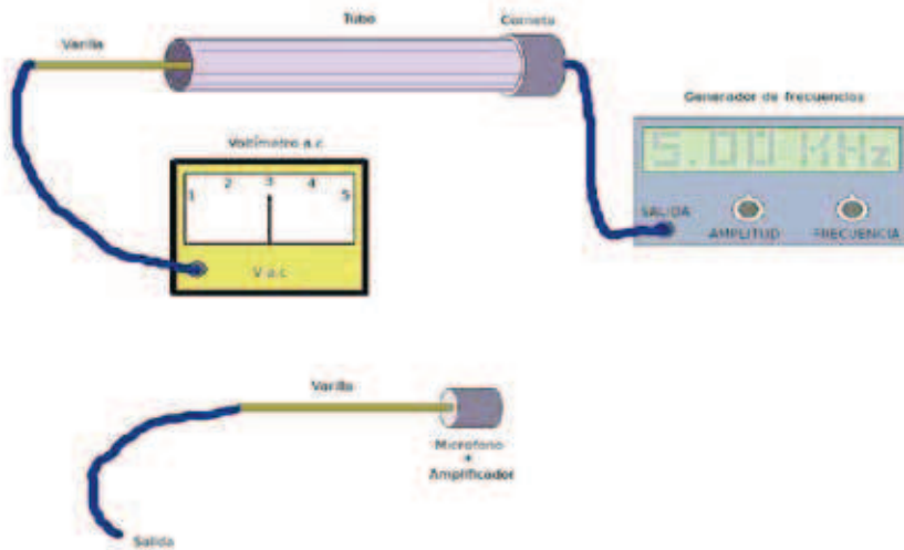
Figura 5. Montaje experimental
